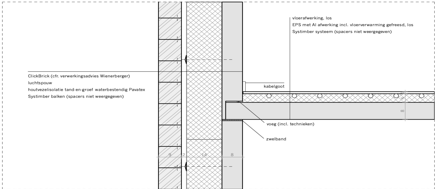
AANSLUITING VERDIEPINGSVLOER
