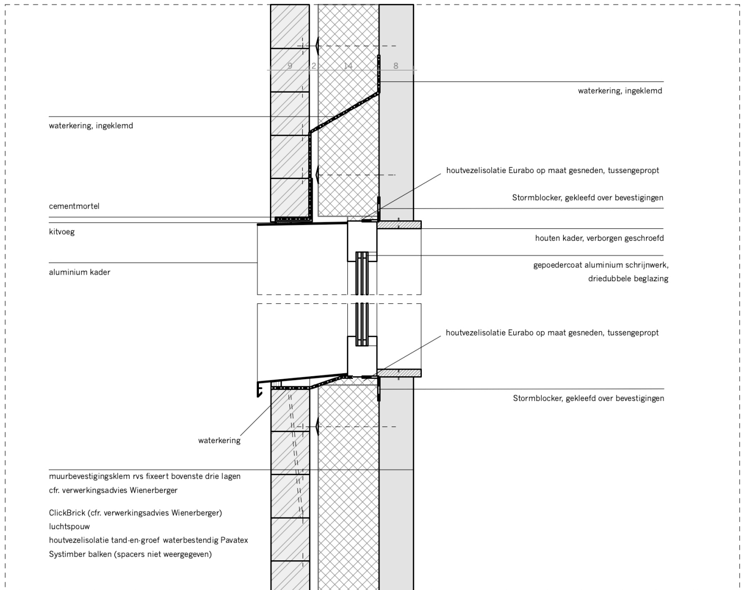
RAAMAANSLUITING
